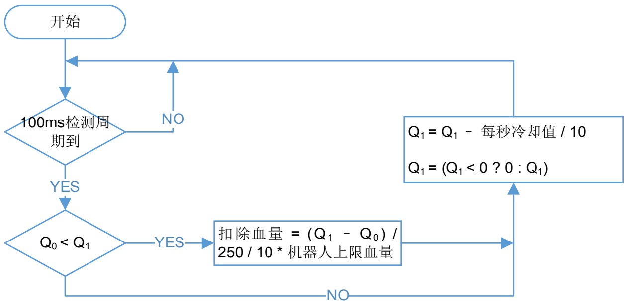
图 3-2 枪口热量超限的扣血逻辑图（上）和冷却逻辑图（下）
