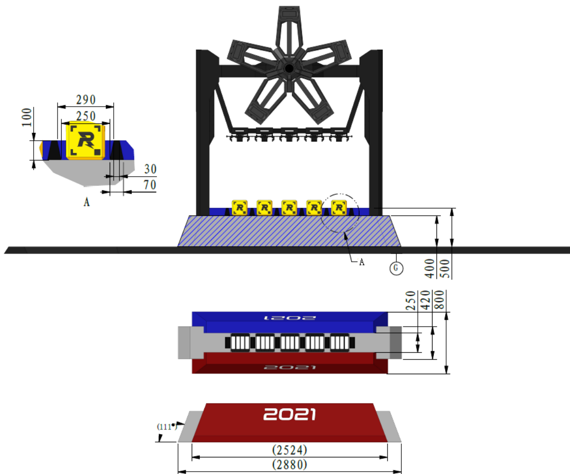
图 4-2 资源岛尺寸示意图
