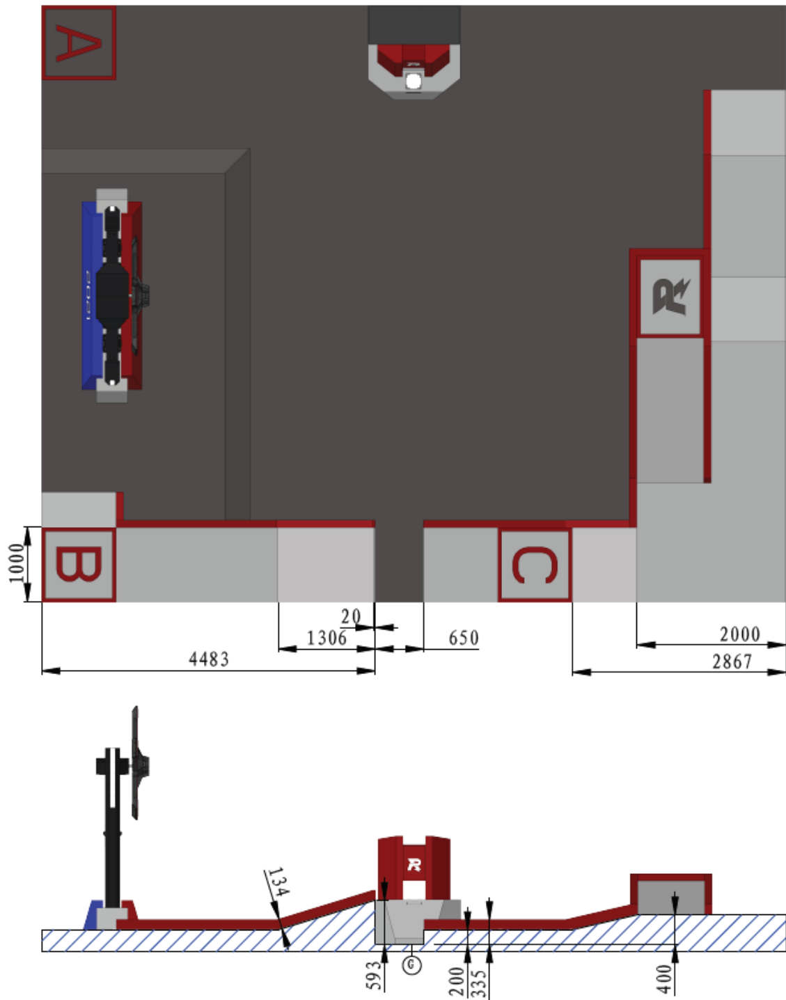
图 4-7 公路示意图
